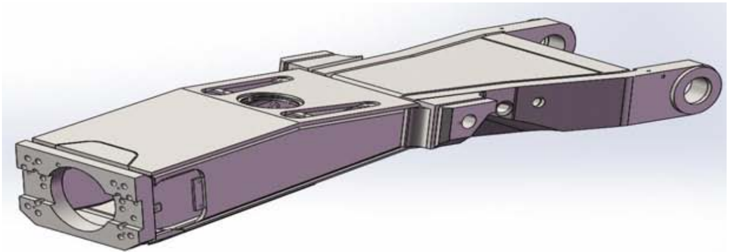
截割大臂/CUTTER BOOM
