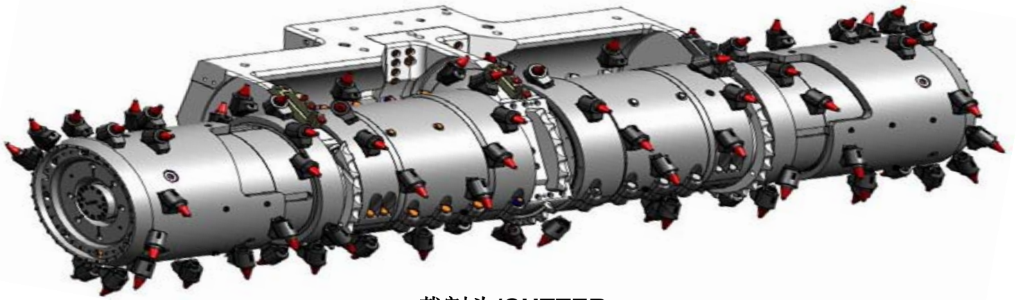
截割头/CUTTER
